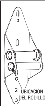
BISAGRA #2 PARA EXTREMO
