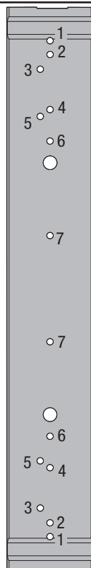
PATRÓN DE AGUJEROS DE LARGUERO DEL EXTREMO (LADO IZQUIERDO. EL LADO DERECHO ES EL LADO OPUESTO.)
