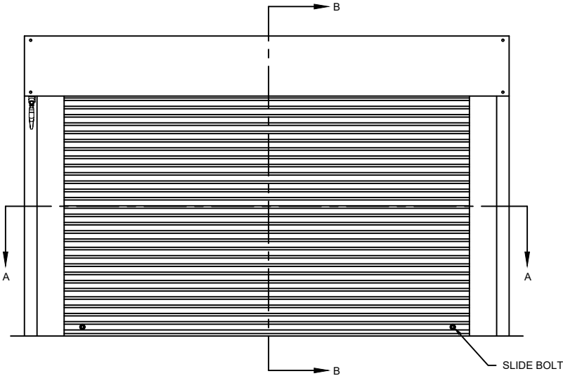
ELEVATION
