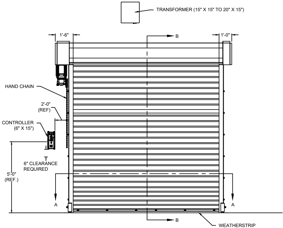
ELEVATION
