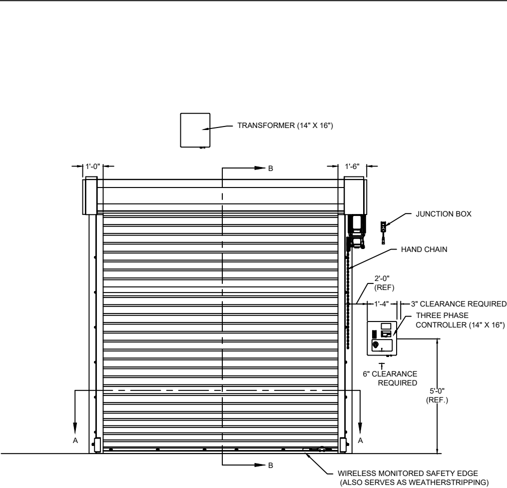
ELEVATION
