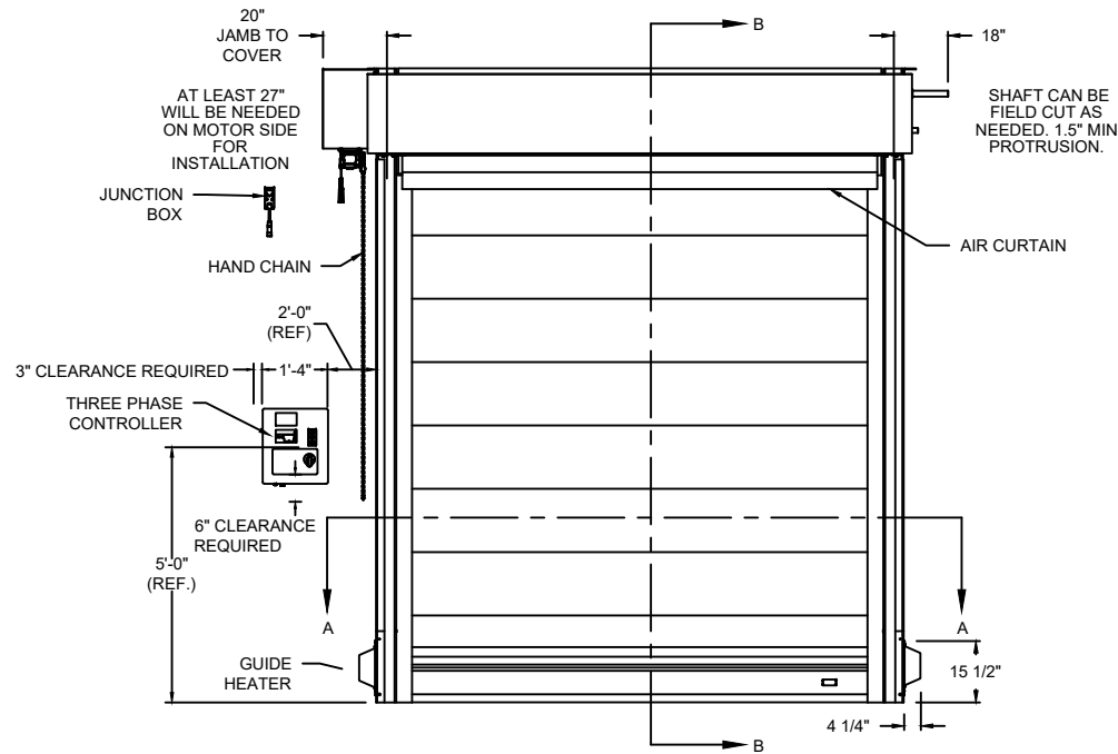
ELEVATION
