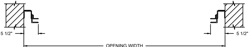
SECTION A-A
