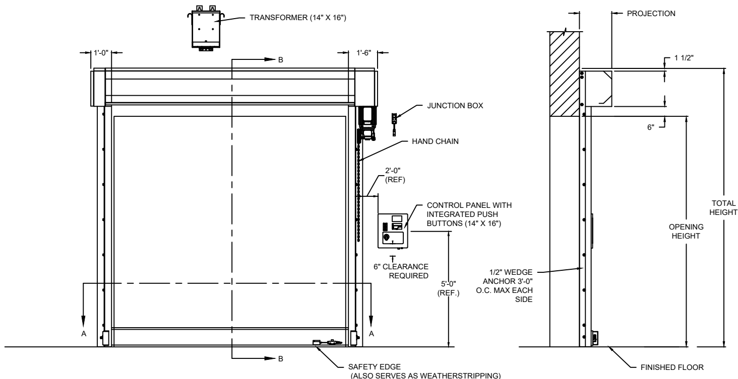
ELEVATION
