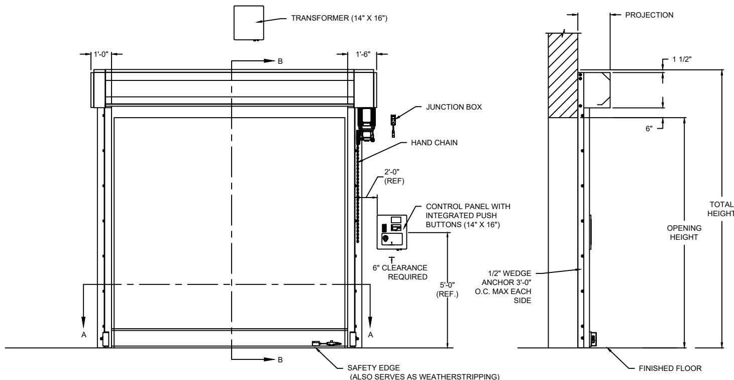
ELEVATION
