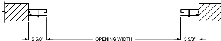
SECTION A-A
