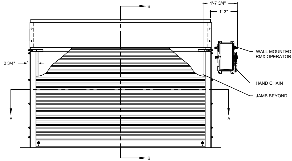
ELEVATION
