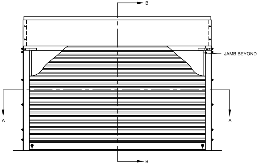
ELEVATION
